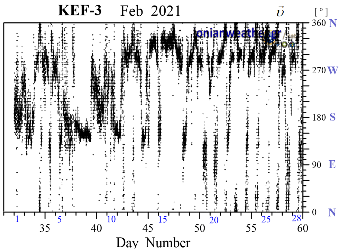
Εικόνα KEF3-3: Μέση ανά λεπτό κατεύθυνση ανέμου Φεβρουαρίου 2021 (κλίμακα αζιμουθίων δεξιά)
