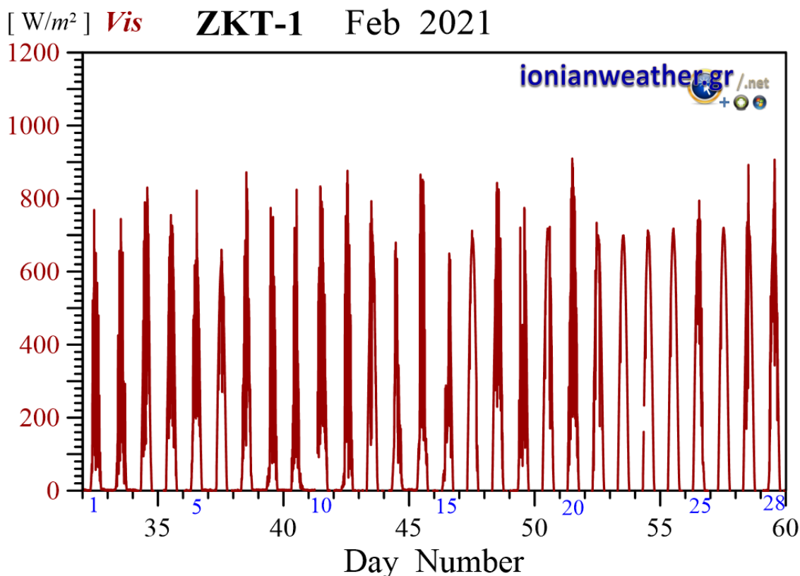
Εικόνα ZKT1-7: Μέση ανά λεπτό Ηλιακή ακτινοβολία Φεβρουαρίου 2021 στην οπτική και εγγύς υπέρυθρη περιοχή.
