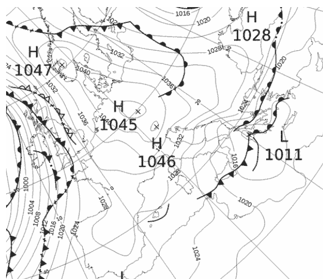
Εικόνα 3.1-14: MSLP 14 February 2021 00UTC
