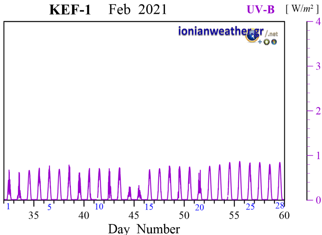
Εικόνα KEF1-9: Μέση ανά λεπτό Ηλιακή ακτινοβολία Φεβρουαρίου 2021 στη φασματική περιοχή UVB
