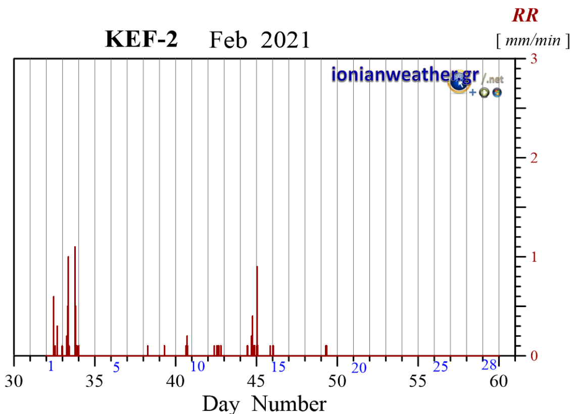
Εικόνα KEF2-1: Ανά λεπτό ρυθμός βροχόπτωσης (mm/min) Φεβρουαρίου 2021.
