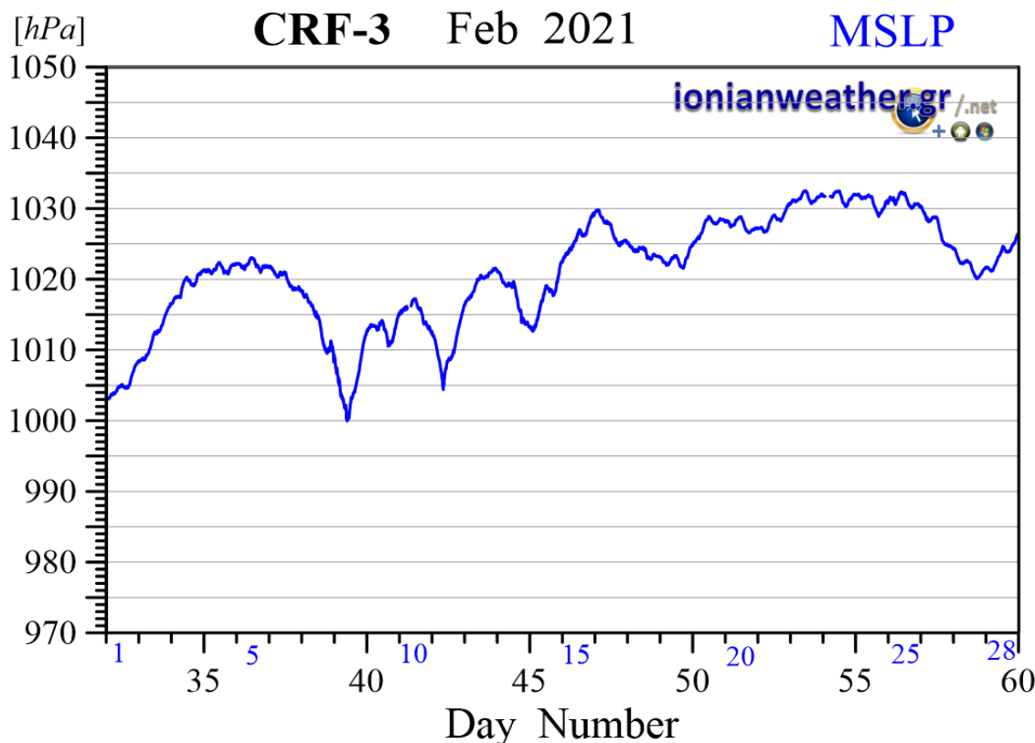
Εικόνα CRF3-6: Μέση ανά λεπτό βαρομετρική πίεση Φεβρουαρίου 2021 ανηγμένη στην επιφάνεια της θάλασσας.
