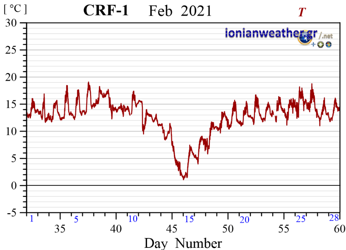
Εικόνα CRF1-4: Μέση ανά λεπτό θερμοκρασία αέρα Φεβρουαρίου 2021.
