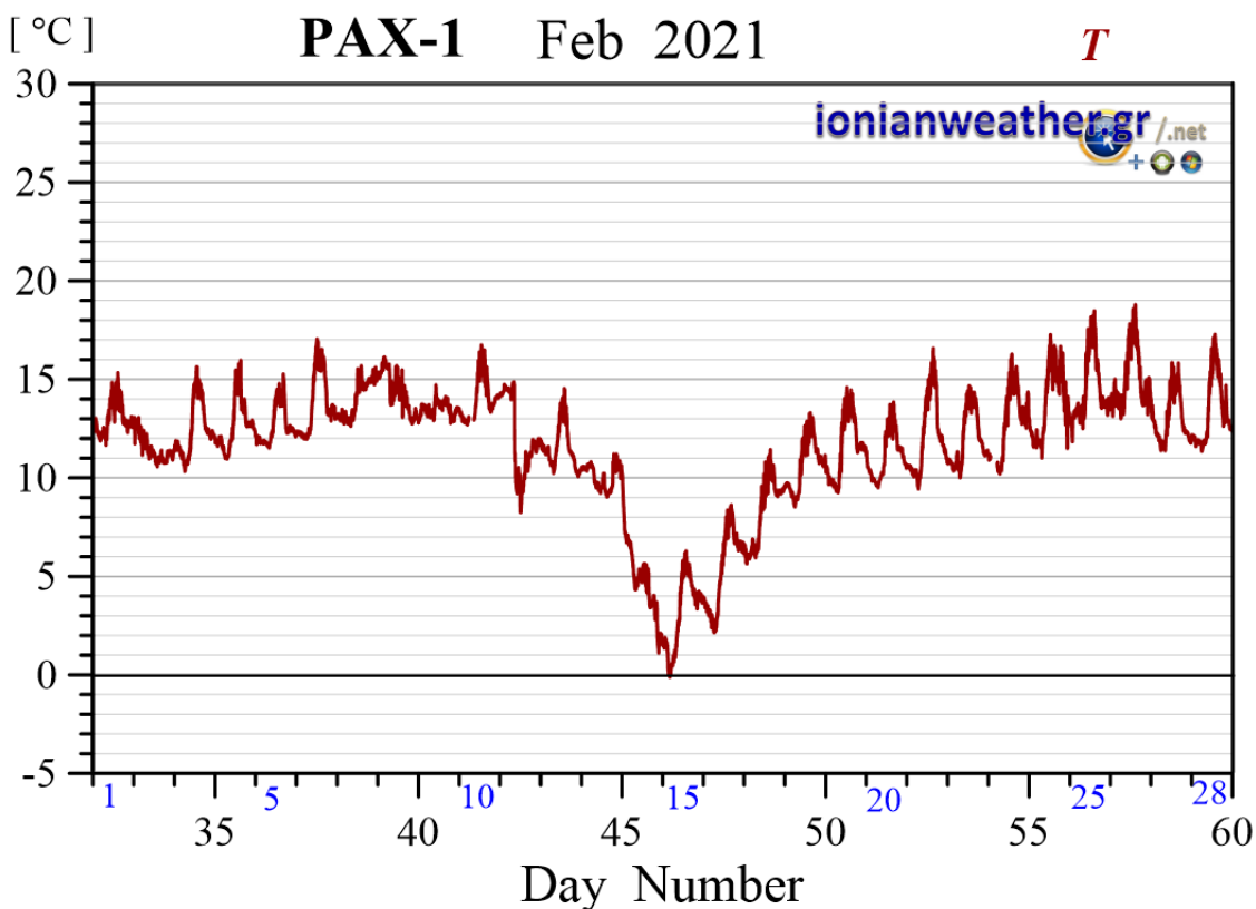
Εικόνα PAX 1-4: Μέση ανά λεπτό θερμοκρασία αέρα Φεβρουαρίου 2021.
