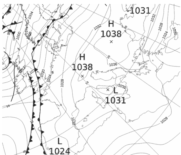
Εικόνα 3.1-25: MSLP 25 February 2021 00UTC
