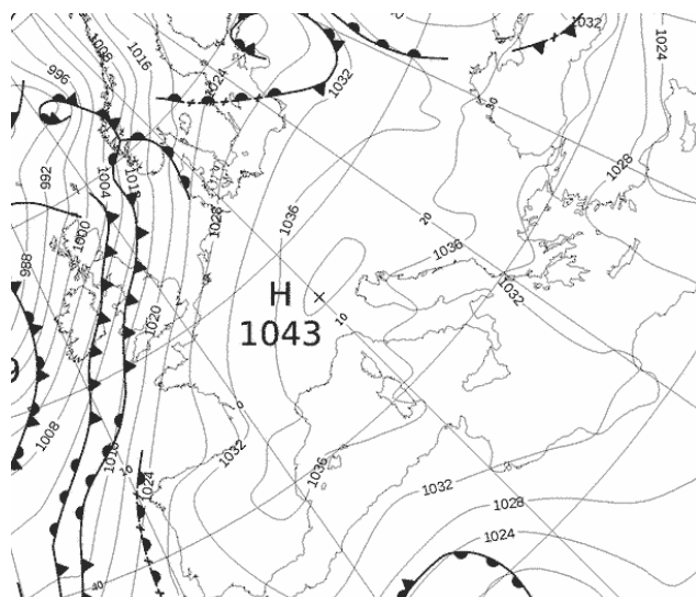
Εικόνα 3.1-24: MSLP 24 February 2021 00UTC
