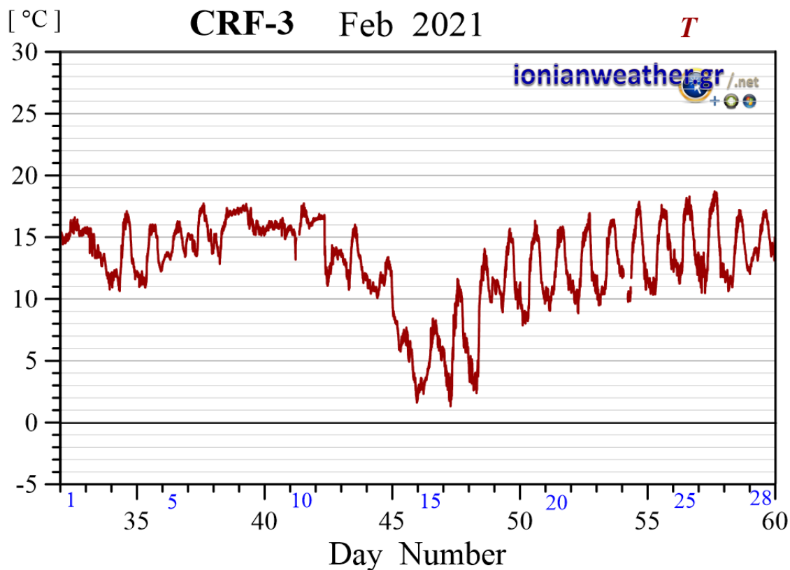
Εικόνα CRF3-4: Μέση ανά λεπτό θερμοκρασία αέρα Φεβρουαρίου 2021.
