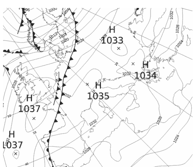
Εικόνα 3.1-26: MSLP 26 February 2021 00UTC
