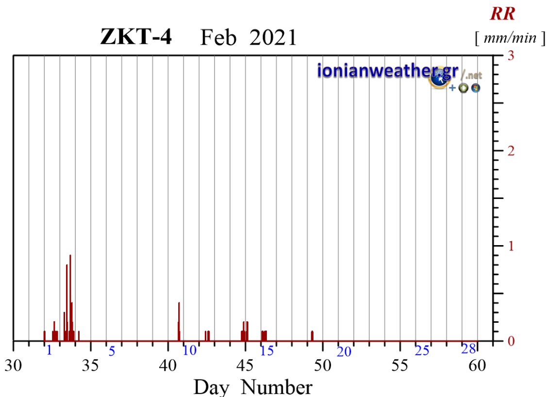
Εικόνα ZKT4-1: Ανά λεπτό ρυθμός βροχόπτωσης (mm/min) Φεβρουαρίου 2021.
