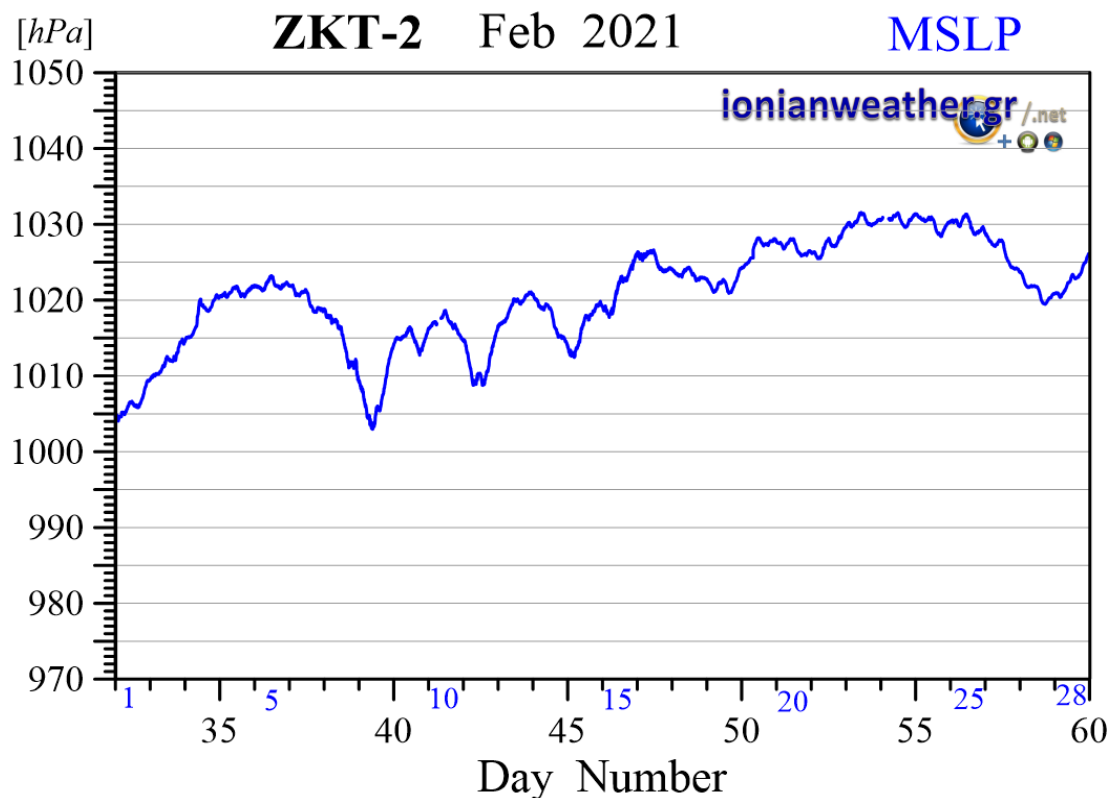
Εικόνα ZKT2-6: Μέση ανά λεπτό βαρομετρική πίεση Φεβρουαρίου 2021 ανηγμένη στην επιφάνεια της θάλασσας.
