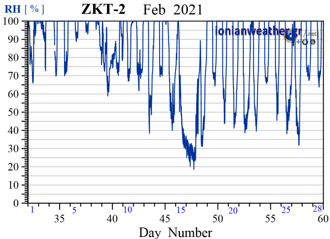
Εικόνα ZKT2-5: Μέση ανά λεπτό σχετική υγρασία Φεβρουαρίου 2021.
