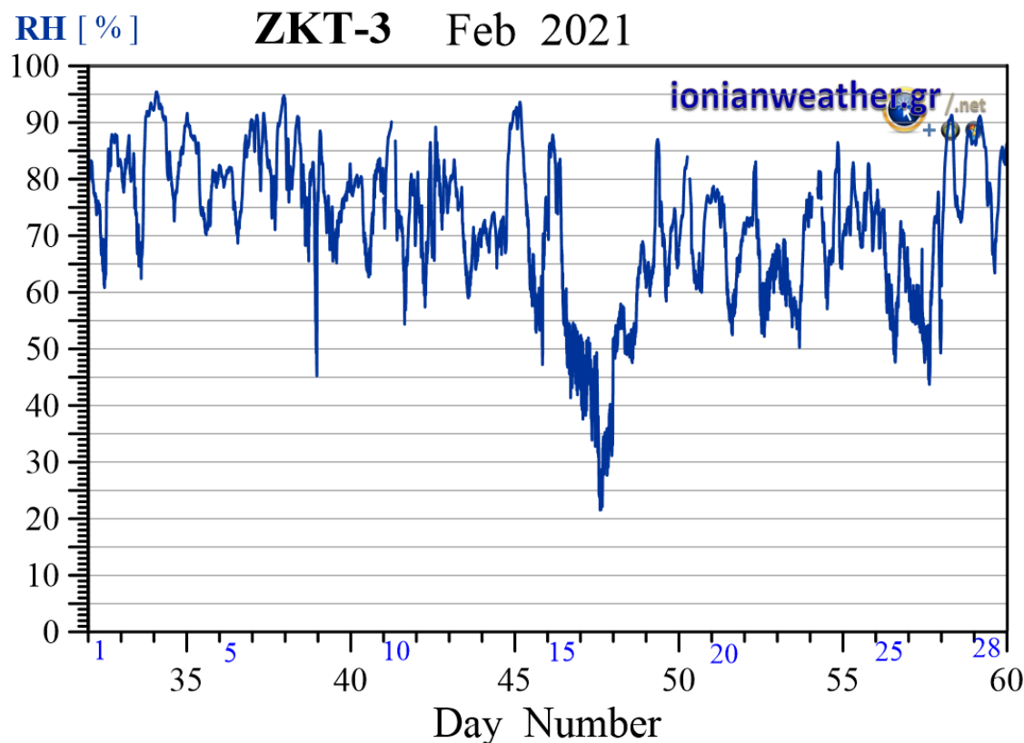
Εικόνα ZKT3-5: Μέση ανά λεπτό σχετική υγρασία Φεβρουαρίου 2021.
